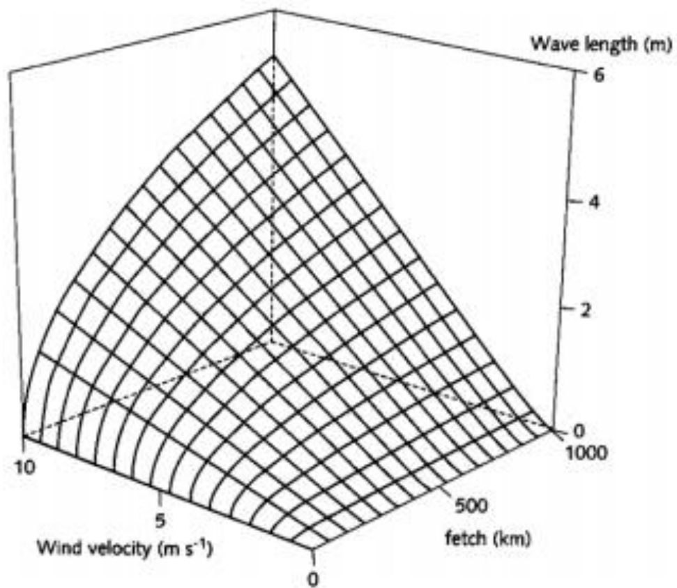
Figuur 7: Invloed van strijklengthe (fetch) en windsnelheid op de golfhoogte. Verkregen via de HAS Hogeschool s'-Hertogenbosch
